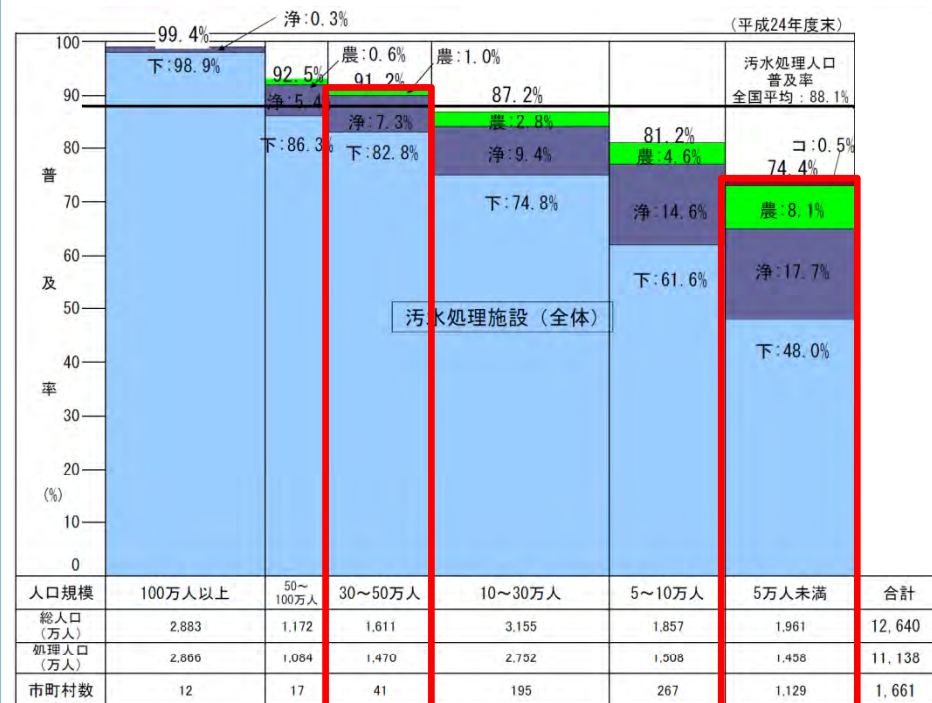
○都市規模別汚水処理人口普及率
